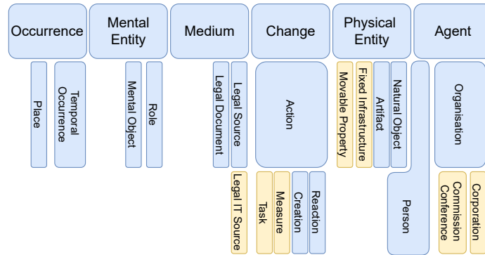
Fig. 3: Entity hierarchy
